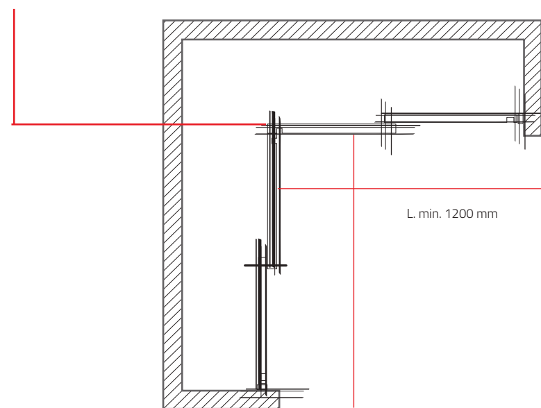
Dettaglio profilo maniglia Ali_Ante per composizioni ad angolo. Detail of Ali_Ante handle profile for corner compositions.
