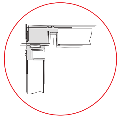
Dettaglio profilo maniglia Ali_Ante per composizioni ad angolo. Detail of Ali_Ante handle profile for corner compositions.
